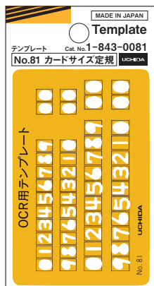
No.1-843-0081 No.81 カードサイズ定規 400円(税込440円) 出荷単位 1枚 材質：塩化ビニール製 本体サイズ： 横55×縦85mm×厚さ0.4mm 文字高：4.5mm・5.5mm
